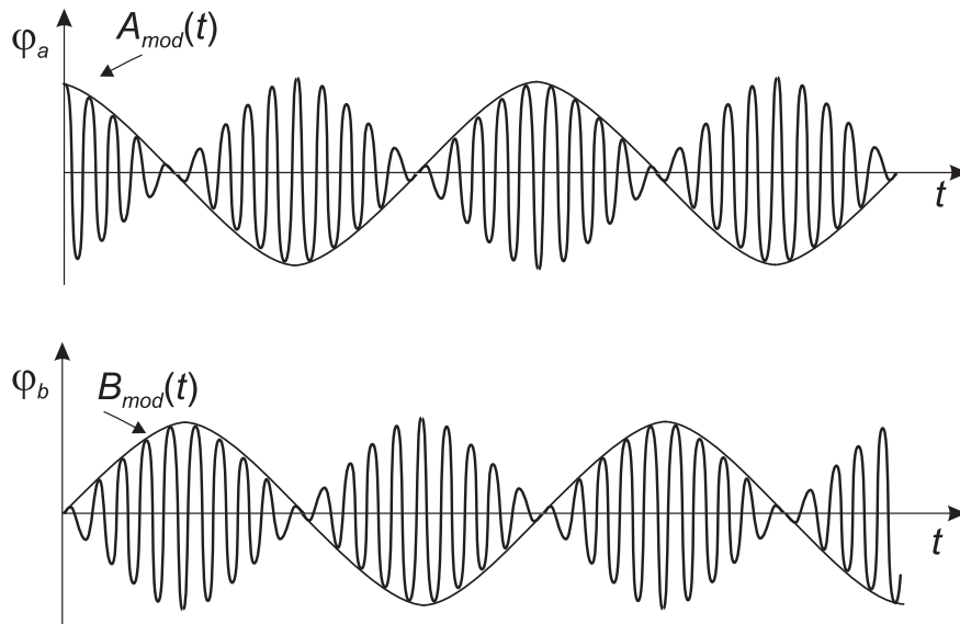
Rysunek 2. Wychylenia \varphi_a(t) i \varphi_b(t) wahadeł sprzężonych wykonujących dudnienia (jednakowe amplitudy drgań normalnych, zerowe fazy początkowe). Źródło: [1].
